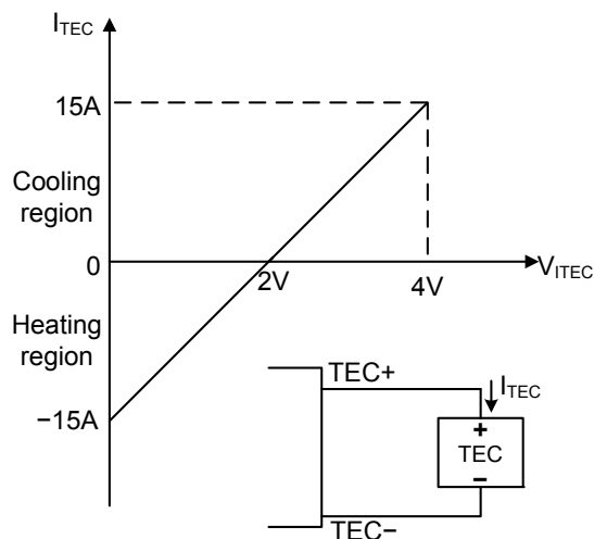
Figure 14. V_{\text{ITEC}} vs. I_{\text{TEC}}
