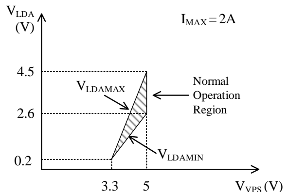
Figure 7. V_{VPS} & V_{LDA}
