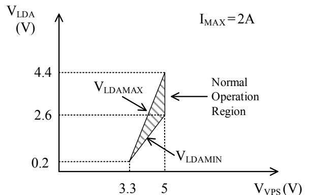
Figure 7. V_{VPS} vs. V_{LDA}
