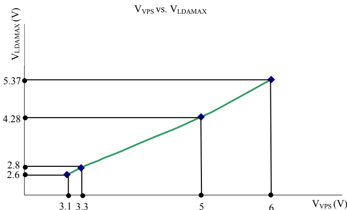
Figure 6. V_{VPS} vs. V_{LDAMAX}
