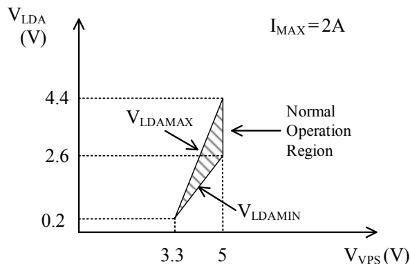
Figure 7. V_{VPS} vs. V_{LDA}
