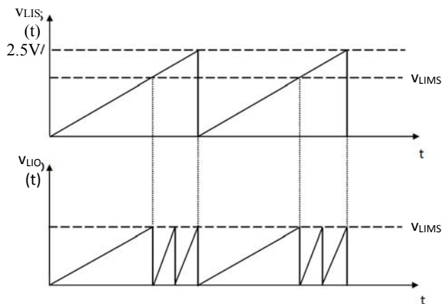
Figure 14. v_{LIS} & v_{LIO}
