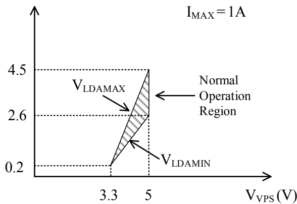
Figure 6. V_{VPS} & V_{LDA}
