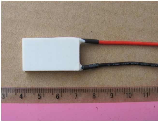
Figure 1. The Photo of Actual ATE1-35
