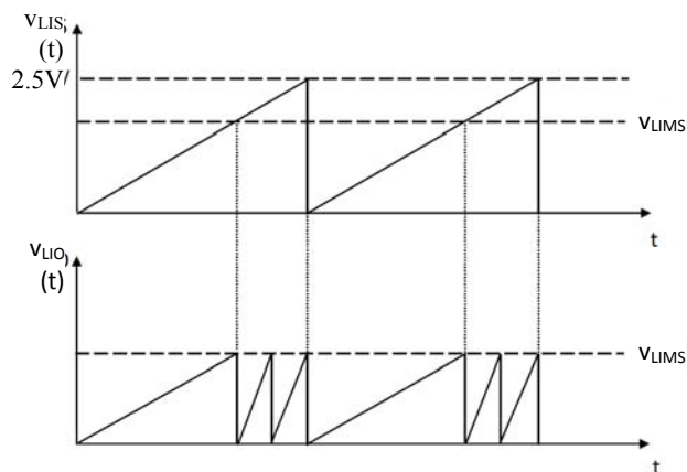
Figure 13. v_{LIS} & v_{LIO}
