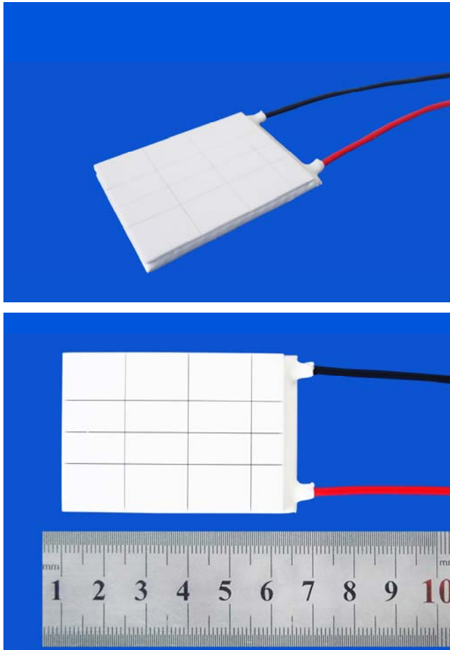
Figure 1. The Photo of Actual ATE1-TC-70-15AS
