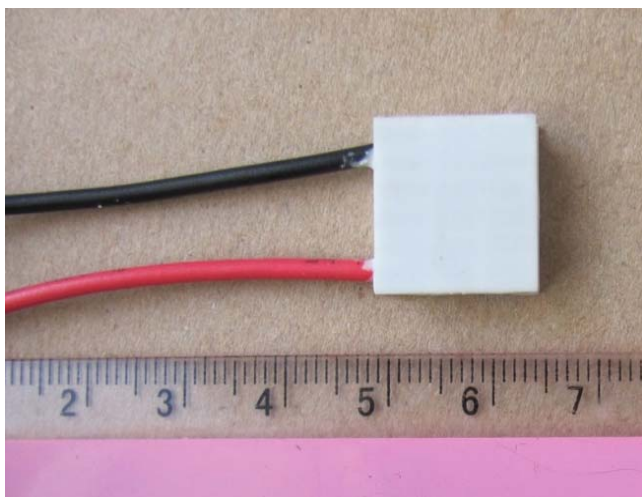
Figure 1.2. The Photo of Actual ATE1-17
