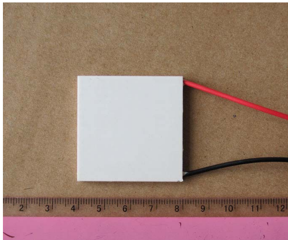
Figure 1.2. The Photo of Actual ATE1-127
