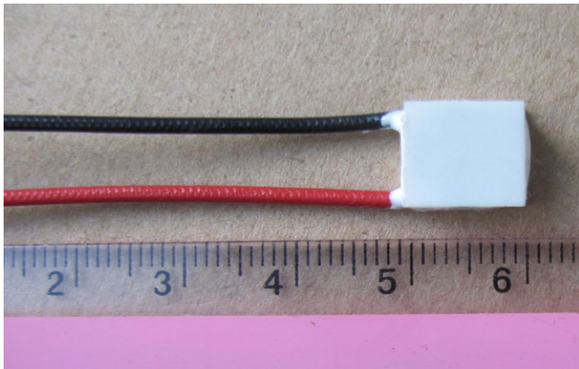
Figure 1.2. The Photo of Actual ATE1-07
